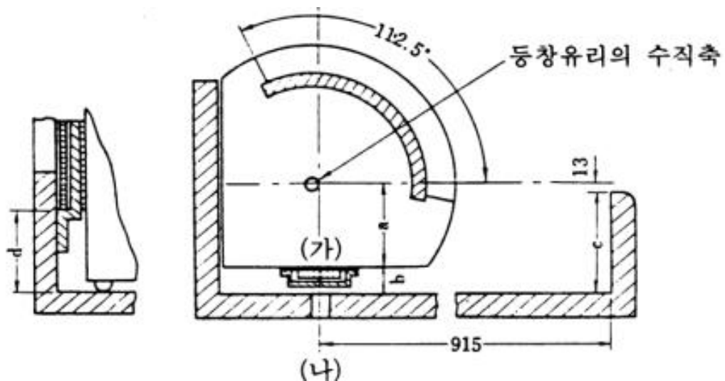
평면도(가)-(나)의 단면도
